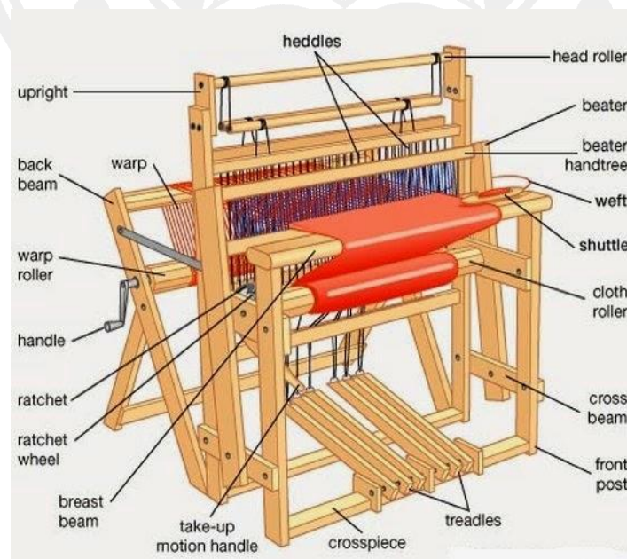
Fig: A basic loom
